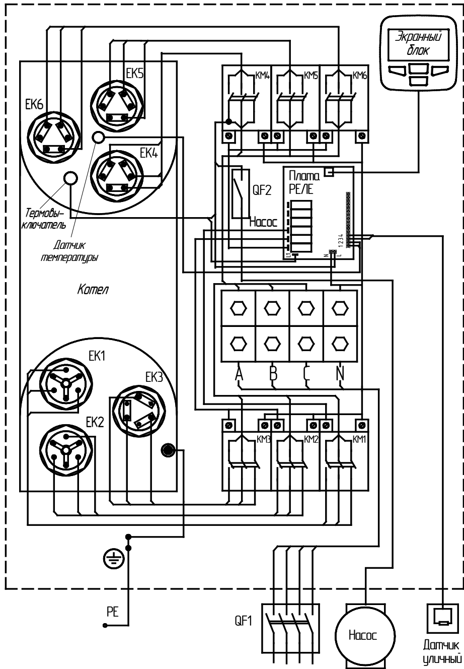
Рисунок 10. Схема подключения ЗВАН UNIVERSAL -72, 90 - 16 -
