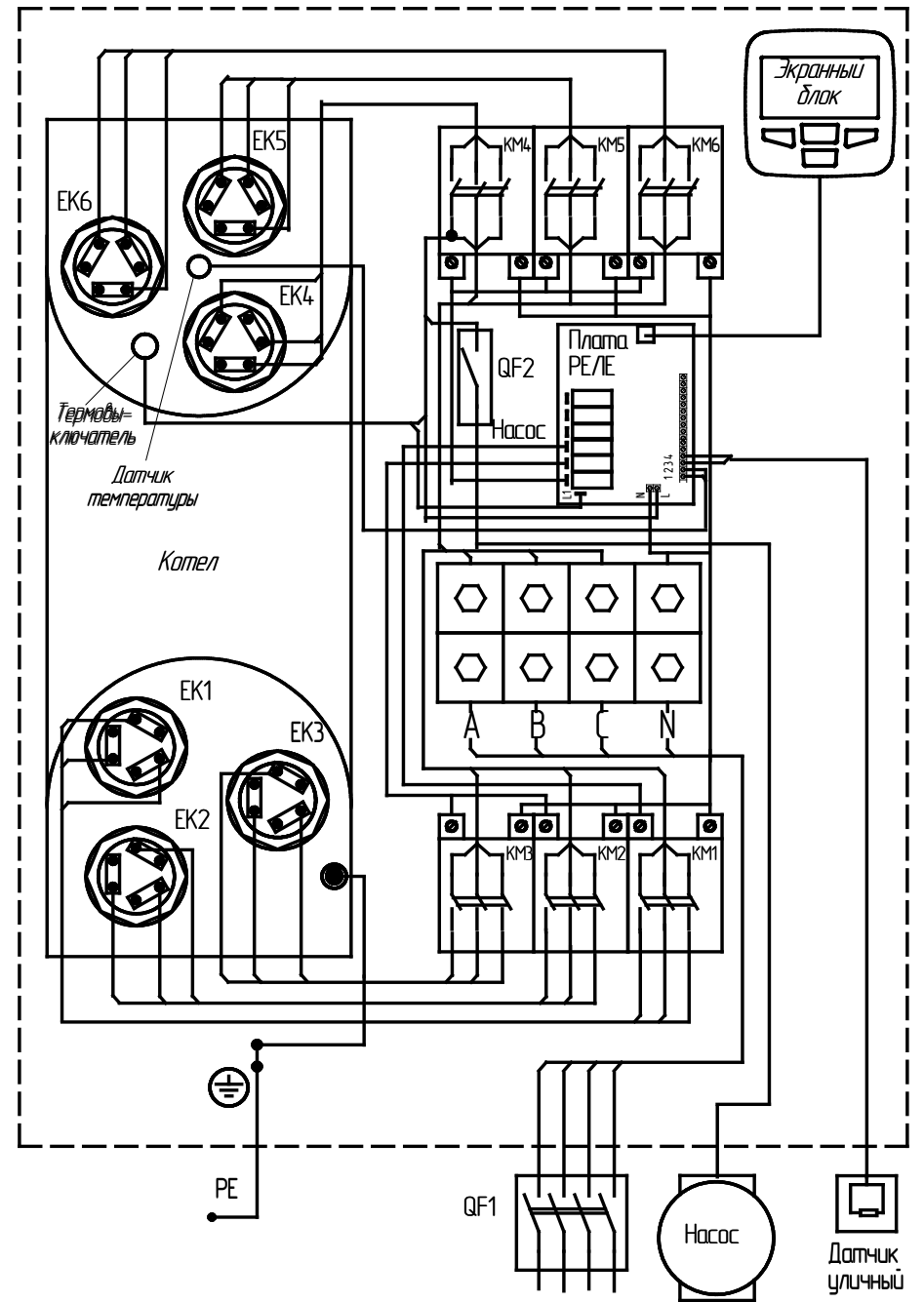
Рисунок 11. Схема подключения ЗВАН UNIVERSAL -81, 96, 105, 120 - 17 -
