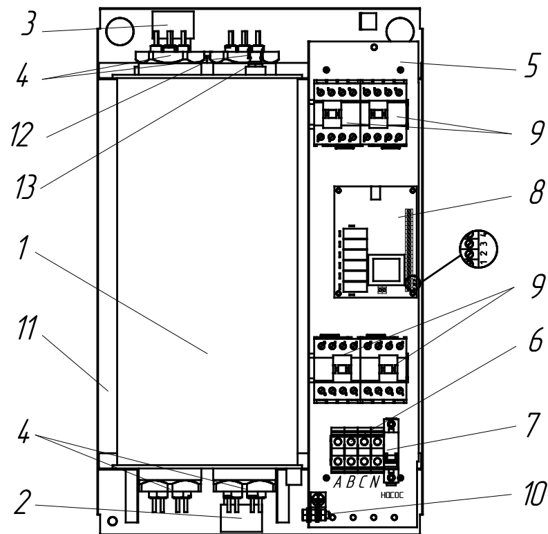
Рисунок 2 Схема внутреннего устройства прибора
