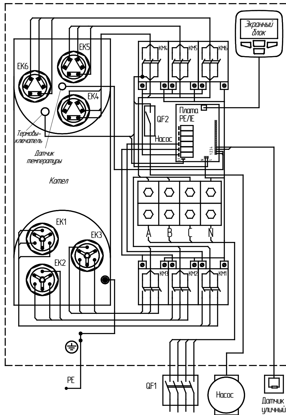
Рисунок 9. Схема подключения ЭВАН UNIVERSAL -66 - 15 -
