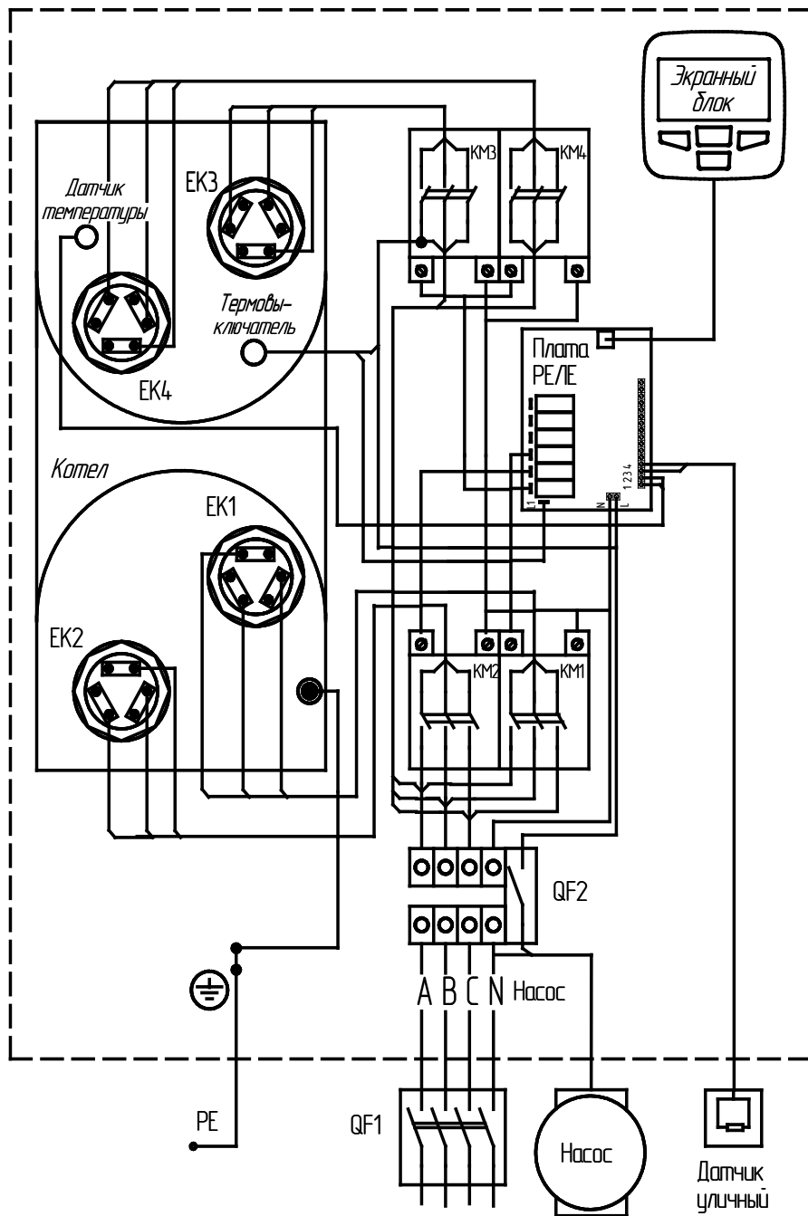
Рисунок 8. Схема подключения ЗВАН UNIVERSAL -60 - 14 -
