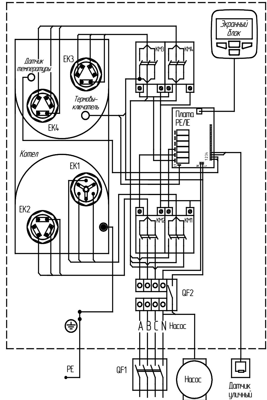
Рисунок 7. Схема подключения ЗБАН UNIVERSAL -4,8, 54 - 13 -
