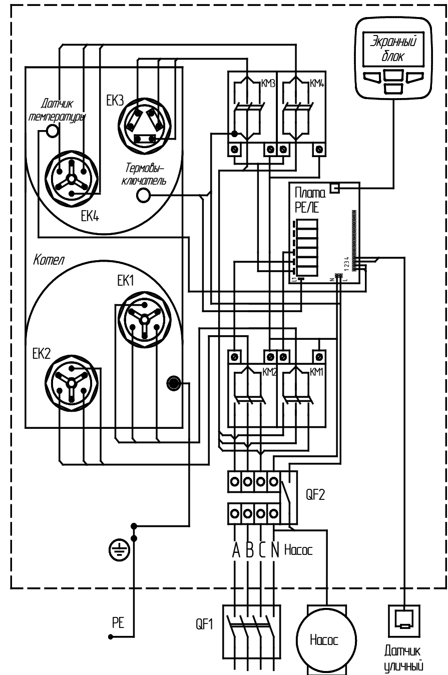
Рисунок 5. Схема подключения ЗВАН UNIVERSAL -36 - 11 -
