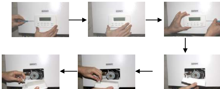
Рисунок 2 Порядок извлечения блока управления.
