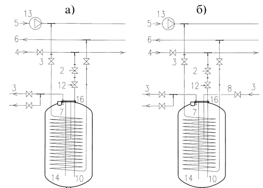
Рис. 5. Схема гидросистемы: а) без циркуляции, б) с циркуляцией 1. воздуховыпускной клапан, 2. редукционный клапан, 3. теплая вода / вход циркуляции, 4. холодная вода, 5. вход теплообменника, 6. выход теплообменника, 7. датчики, 8. циркуляция, 9. водосливной вентиль, 10. элевик-теплообменник, 11. ТЭН, 12. предохранительный клапан, 13. циркуляционный насос, 14. трубка РEX, 15. тройник, 16. крышка
