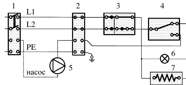
3 Электросхема
